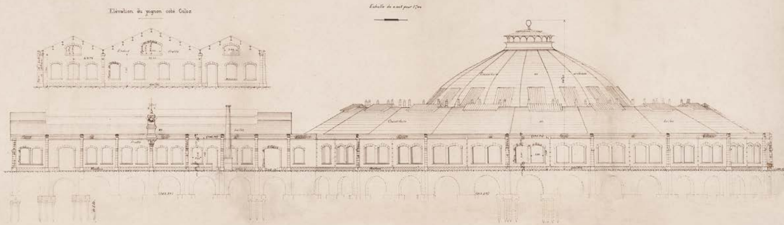
Élévation de l'atelier de levage et de la rotonde suivant AB du plan
